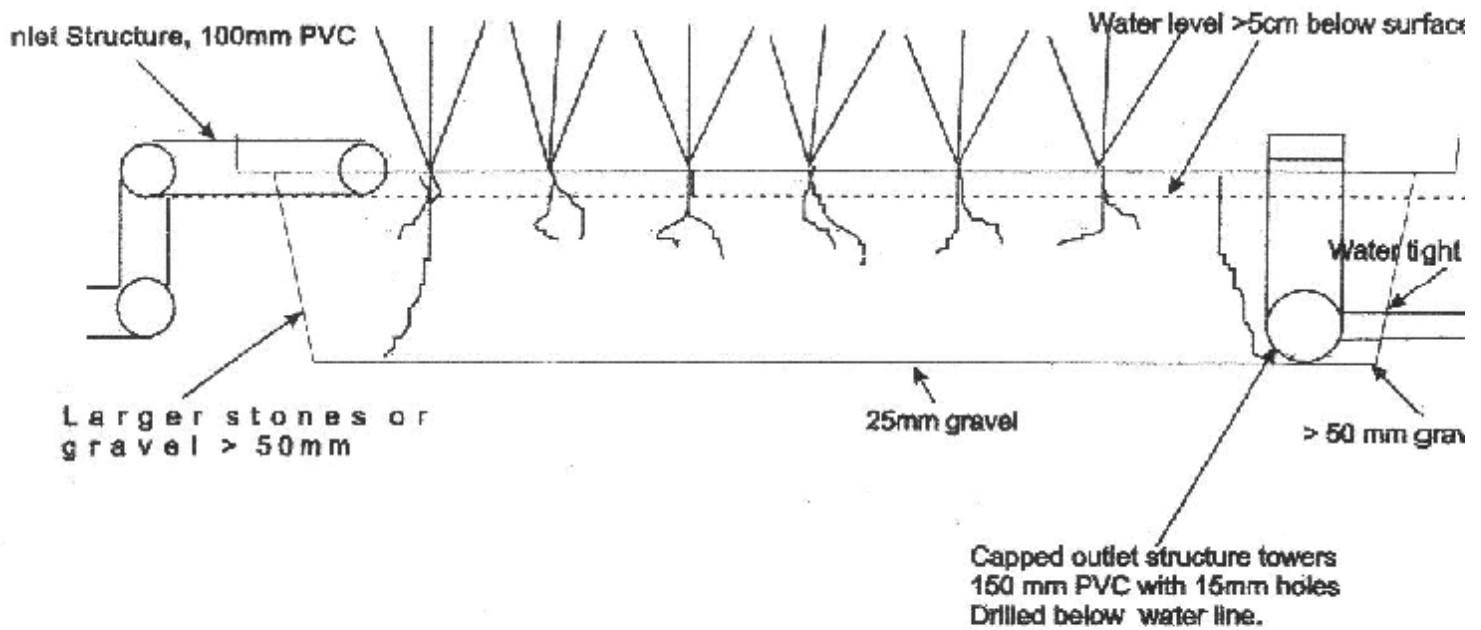
Elevation
